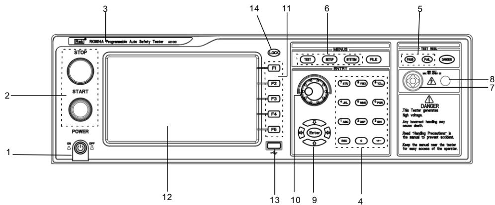
图 3-1 前面板说明
